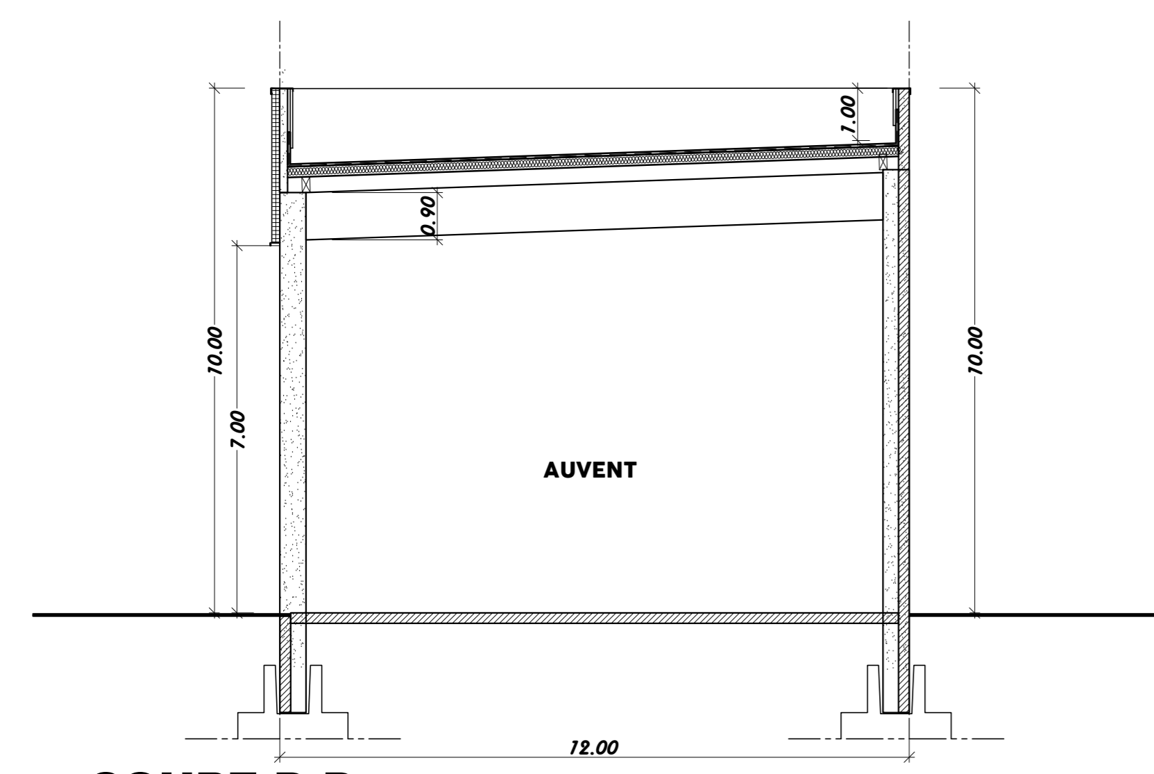
COUPE D.D.
